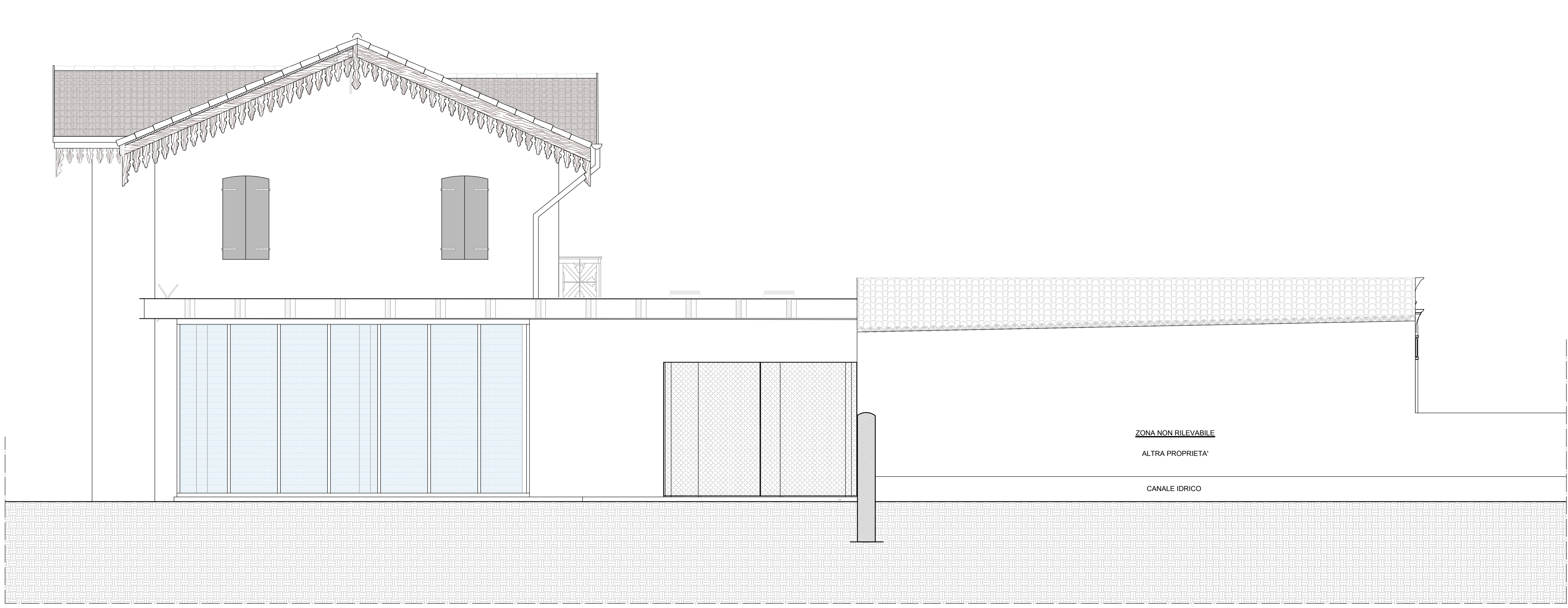
PROSPETTO NORD
