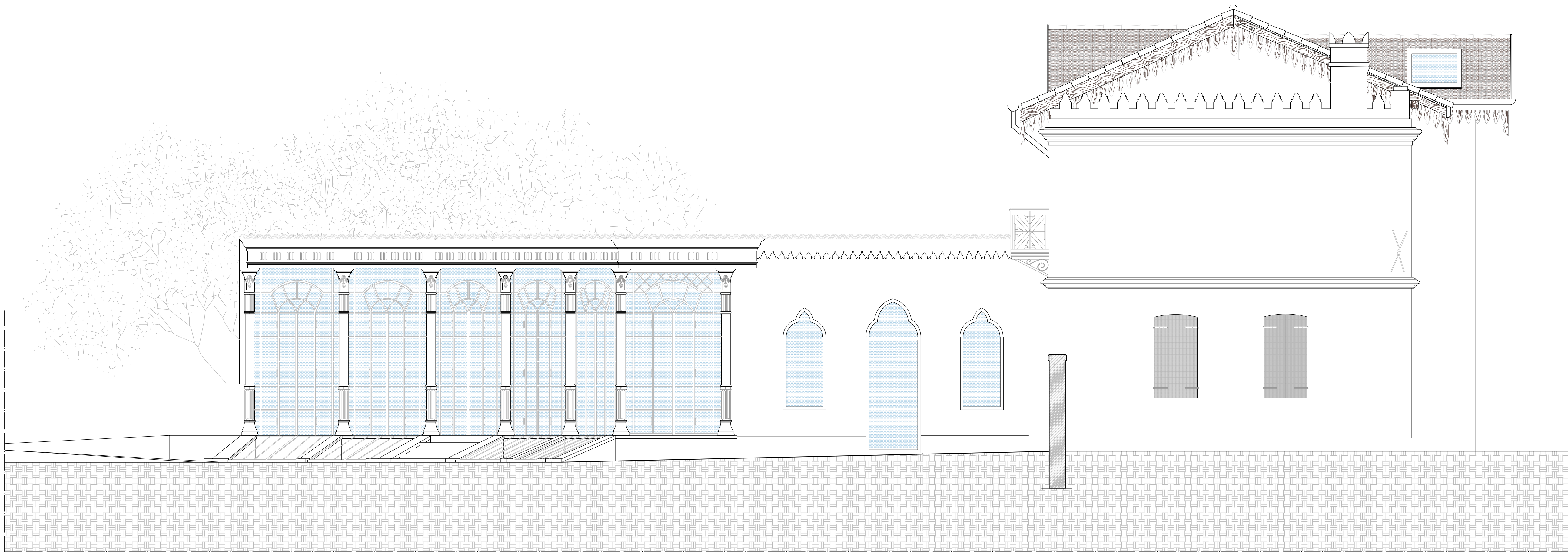
PROSPETTO SUD
